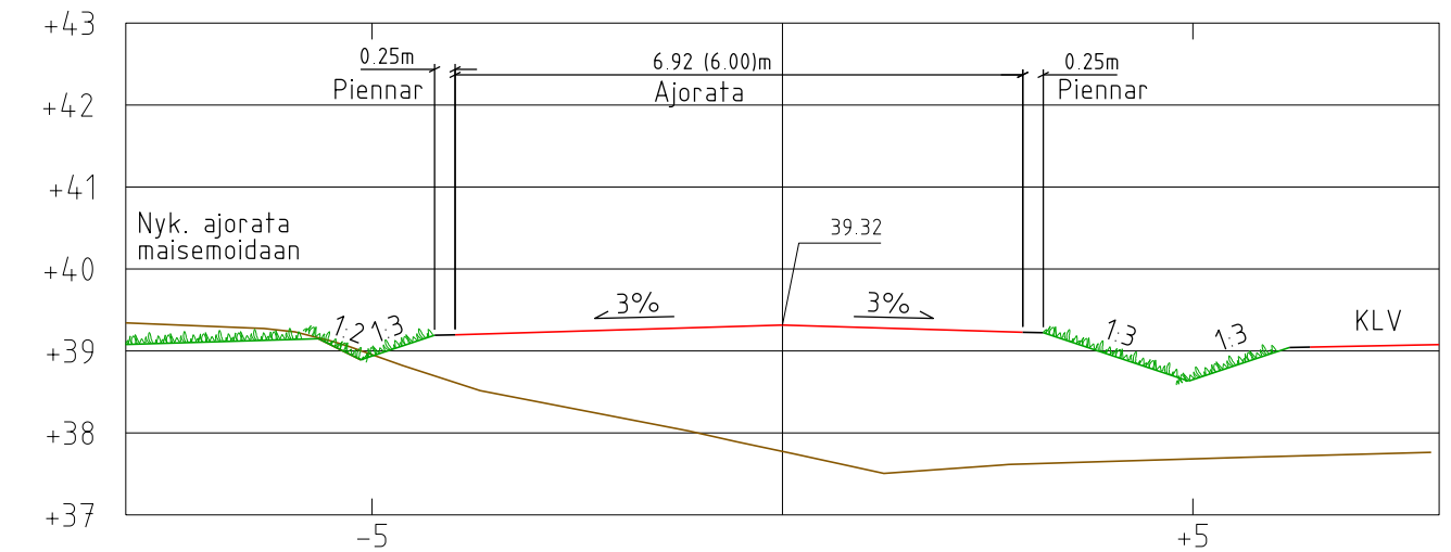
Tyyppipoikkileikkaus 1:100 Paalu 60
