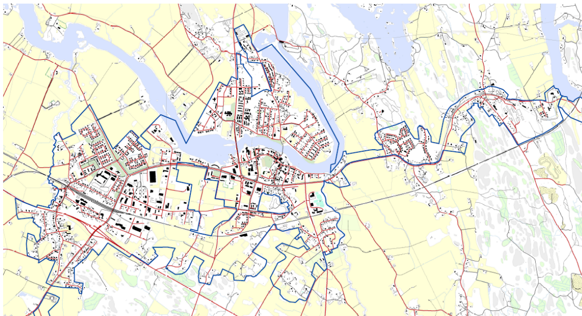
Kuva 43. Vesihuoltoverkoston toiminta-alue Peipohja-Tulkila-Riste
